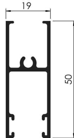
COD: RA 1/902 DINTEL UMBRAL PESO: 0,456 Kg/m LARGO: 6030 mm.
