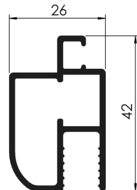
COD: RA 3/035 PARANTE CENTRAL CORREDIZA PESO: 1,531 Kg/m LARGO: 6200 mm.
