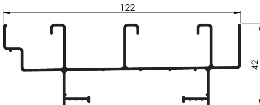
COD: RA 1/862 MARCO TRES GUIAS PESO: 1,160 Kg/m LARGO: 6150 mm.
