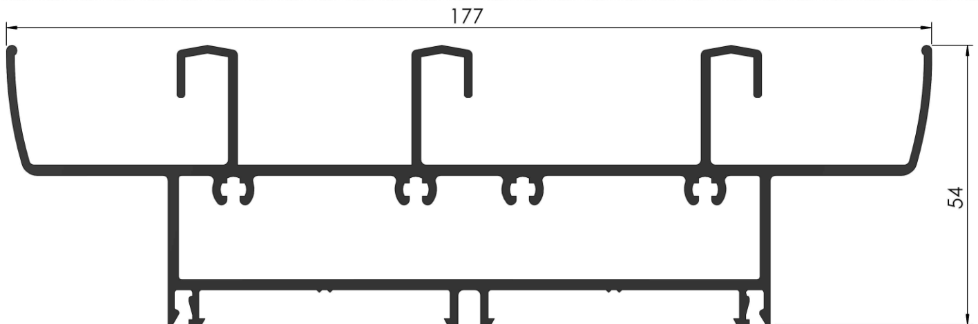
COD: RA 3/081 UMBRAL Y DINTEL CORREDIZA DE 3 HOJAS PESO: 2,908 Kg/m LARGO: 6200 mm.
