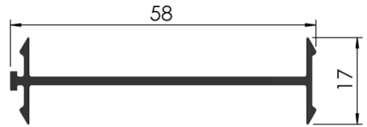
COD: RA 3/067 PERFIL DE ACOPLE PESO: 0,329 Kg/m LARGO: 6200 mm.
