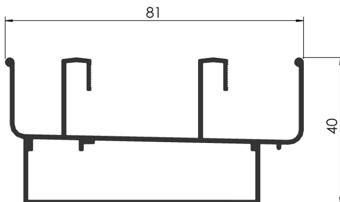
COD: RA / 263 MARCO CORREDIZA PESO: 0,974 Kg/m LARGO: 6030 mm.
