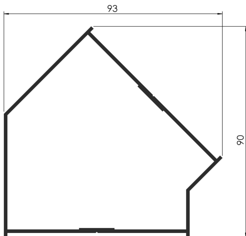
COD: RA 2/184 COLUMNA 45° PESO: 1,120 Kg/m LARGO: 6150 mm.
