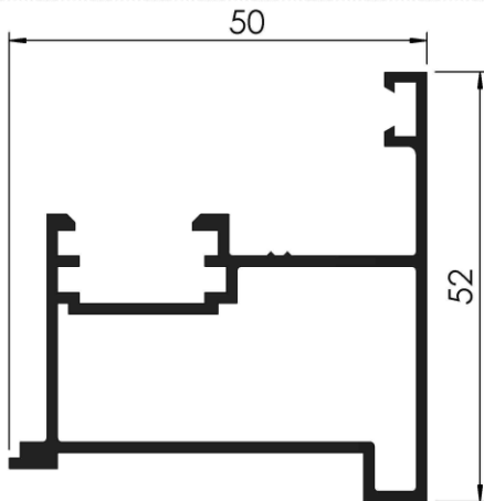
COD: RA 3/224 ENCUENTRO CENT. VENTANA DE ABRIR 2 HOJAS PUERTA DE REBATIR PESO: 0,745 Kg/m LARGO: 6200 mm.
