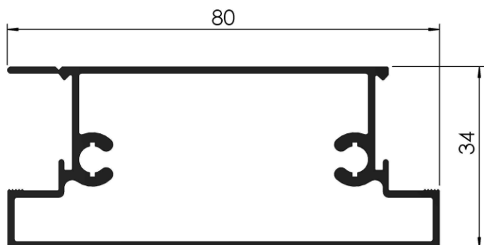
COD: RA 1/941 DINTEL UMBRAL 36 MM. PESO: 0,989 Kg/m LARGO: 6030 mm.
