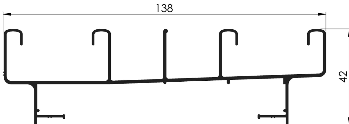
COD: RA 1/864 MARCO CUATRO GUIAS PESO: 1,101 Kg/m LARGO: 6030 mm.
