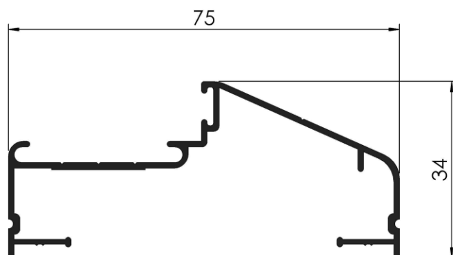
COD: RA 1/193 MARCO PUERTA 36 mm. PESO: 0,530 Kg/m LARGO: 6200 mm.
