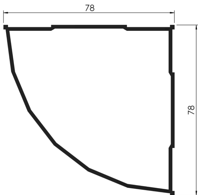
COD: RA 2/184 COLUMNA 45° PESO: 1,120 Kg/m LARGO: 6150 mm.
