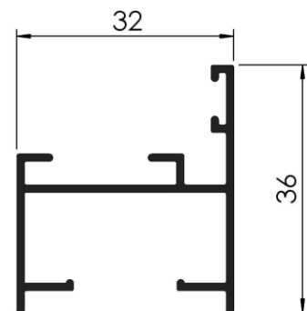
COD: RA 1/577 MARCO ANGOSTO 25 mm. PESO: 0,367 Kg/m LARGO: 6200 mm.
