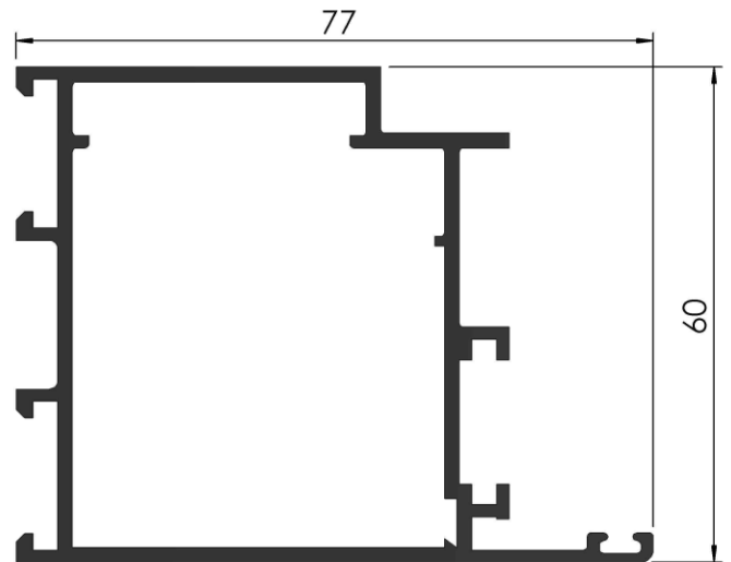
COD: RA 3/041 HOJA PUERTA DE REBATIR PESO: 1,388 Kg/m LARGO: 6200 mm.
