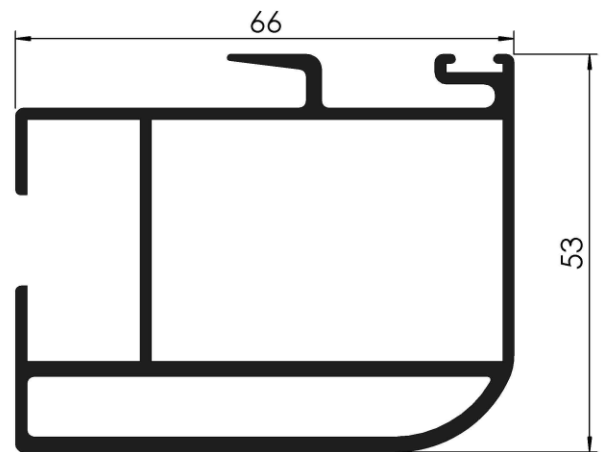
COD: RA 3/035 PARANTE CENTRAL CORREDIZA PESO: 1,531 Kg/m LARGO: 6200 mm.
