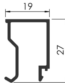
COD: RA 3/046 CONTRAVIDRIO RECTO P/DVH PESO: 0,259 Kg/m LARGO: 6200 mm.
