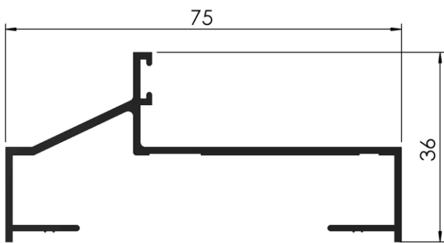
COD: RA 1/479 MARCO DE PUERTA PLACA DE 2" PESO: 0,550 Kg/m LARGO: 6200 mm.
