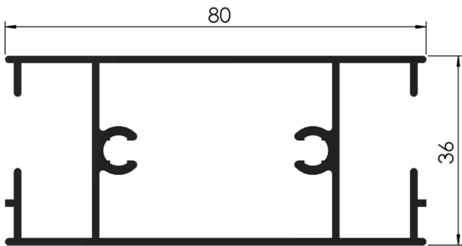
COD: RA 1/180 TRAVESAÑO PUERTA DE REBATIR 36 mm. PESO: 0,980 Kg/m LARGO: 6030 mm.
