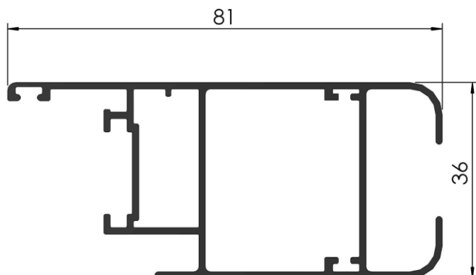
COD: RA / 261 HOJA CORREDIZA PESO: 0,673 Kg/m LARGO: 6030 mm.
