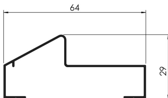
COD: RA H 1/479 MARCO DE PUERTA PLACA PESO: 0,328 Kg/m LARGO: 6200 mm.
