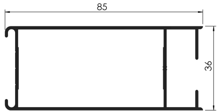
COD: RA 1/179 PARANTE PUERTA DE REBATIR 36 MM. PESO: 0,980 Kg/m LARGO: 6200 mm.
