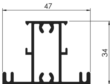
COD: RA 1/777 TRAVESAÑO INTERMEDIO DE PAÑO FIJO PESO: 0,690 Kg/m LARGO: 6030 mm.
