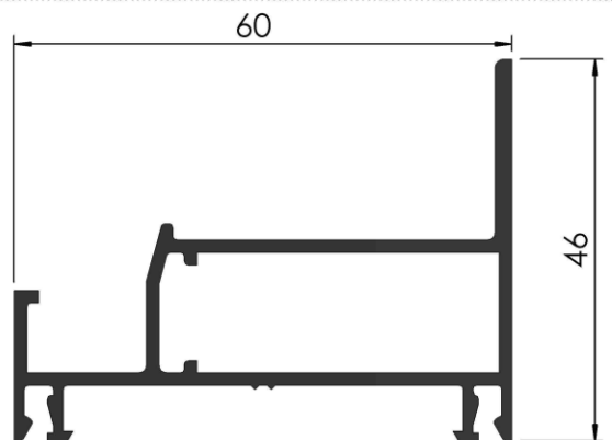
COD: RA 3/067 PERFIL DE ACOPLE PESO: 0,329 Kg/m LARGO: 6200 mm.
