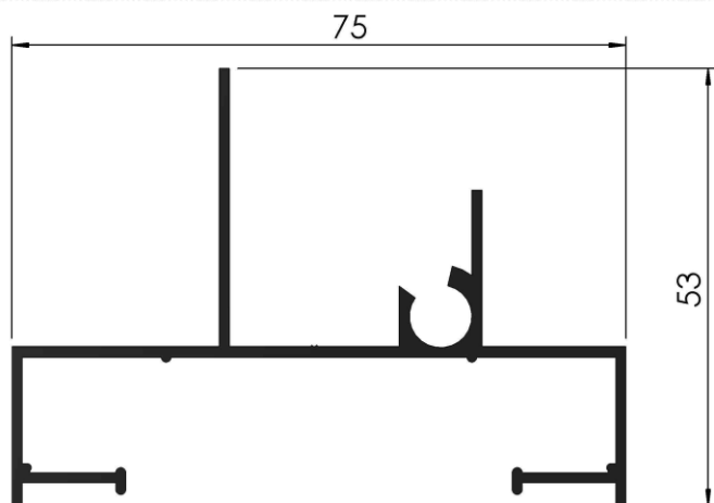
COD: RA 1/014 MARCO PROYECTANTE Y BANDEROLA PESO: 0,810 Kg/m LARGO: 6030 mm.
