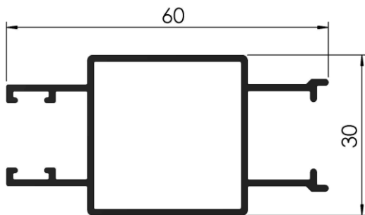
COD: RA 1/053 PARANTE LATERAL REFORZADO DE HOJA CORREDIZA PESO: 0,695 Kg/m LARGO: 6150 mm.
