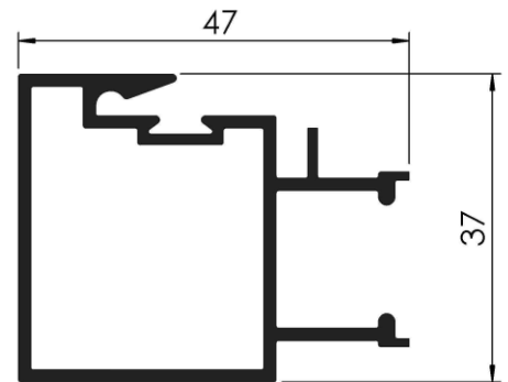
COD: RA 1/054 PARANTE CENTRAL REFORZADO DE HOJA CORREDIZA PESO: 0,720 Kg/m LARGO: 6150 mm.
