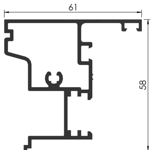
COD: RA 3/053 ENCUENTRO CENTRAL VENTANA DE ABRIR PESO: 1,094 Kg/m LARGO: 6200 mm.
