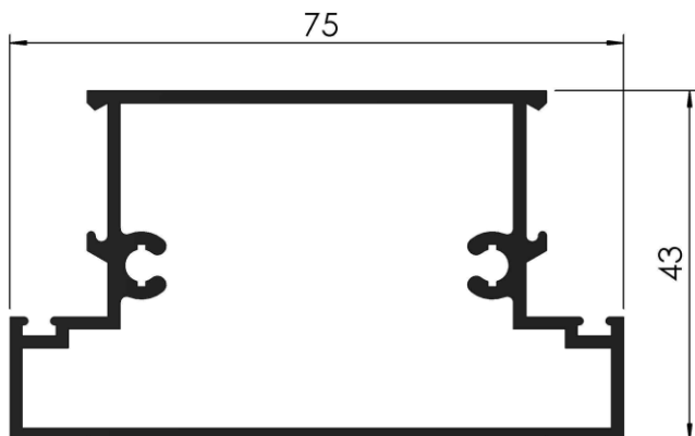
COD: RA 1/616 PARANTE PUERTA 45 mm. PESO: 1,240 Kg/m LARGO: 6200 mm.
