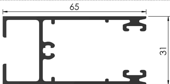
COD: RA 3/061 ZOCALO Y CABEZAL VENTANA CORREDIZA PESO: 0,942 Kg/m LARGO: 6200 mm.
