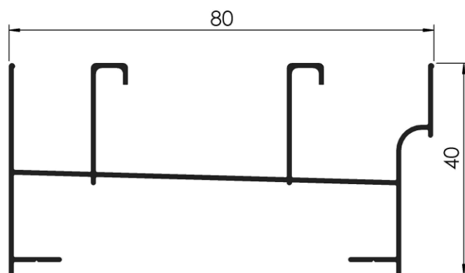
COD: RA E 1/901 MARCO CORREDIZO ECONAL PESO: 0,580 Kg/m LARGO: 6150 mm.
