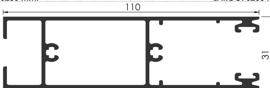
COD: RA 3/062 ZOCALO ALTO PUERTA CORREDIZA PESO: 1,477 Kg/m LARGO: 6200 mm.
