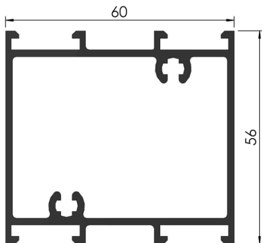
COD: RA 3/042 TRAVESAÑO PUERTA DE REBATIR PESO: 1,399 Kg/m LARGO: 6200 mm.
