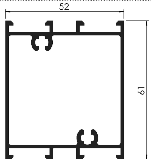
COD: RA 3/218 TRAVESAÑO HOJA PUERTA DE REBATIR PESO: 1,161 Kg/m LARGO: 6030 mm.
