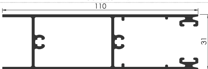
COD: RA 3/074 ZOCALO ALTO CORREDIZA P/DVH PESO: 1,412 Kg/m LARGO: 6200 mm.
