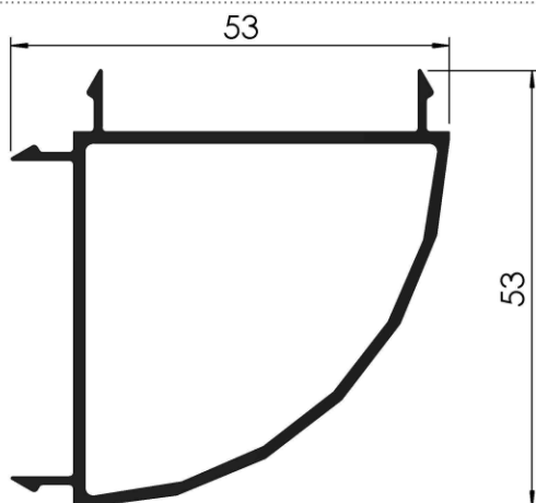
COD: RA 3/262 COLUMNA DE ACOPLE 90° PESO: 0,700 Kg/m LARGO: 6150 mm.
