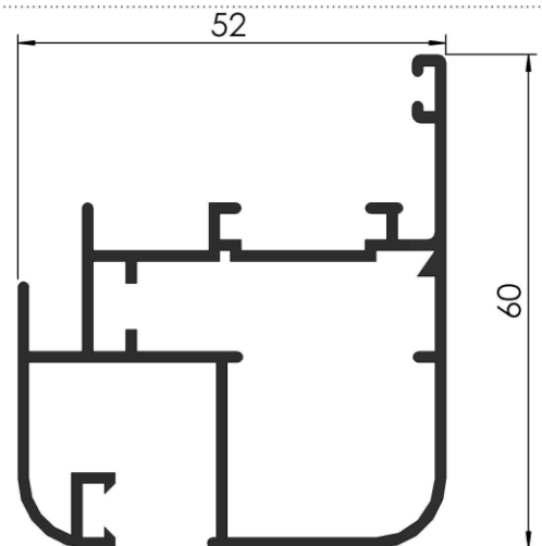
COD: RA 2/235 HOJA DE ABRIR UNIFICADA MODENA PESO: 1,030 Kg/m LARGO: 6030 mm.
