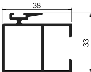
COD: RA 1/204 PARANTE CENTRAL HOJA VENTANA Y PUERTA CORREDIZA 90° PESO: 0,600 Kg/m LARGO: 6150 mm.
