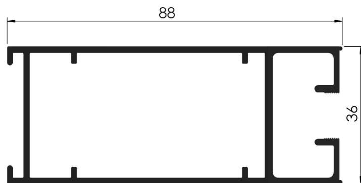
COD: RA 1/938 PARANTE ANCHO 36 mm. PESO: 1,153 Kg/m LARGO: 6200 mm.
