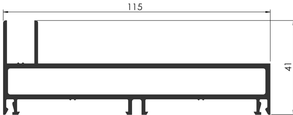
COD: RA 3/080 JAMBA DE MARCO CORREDIZA DE 3 HOJAS PESO: 1,701 Kg/m LARGO: 6200 mm.
