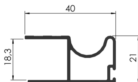
COD: RA / 2 MANIJA TIRADOR PLACARD PESO: 0,431 Kg/m LARGO: 6030 mm.
