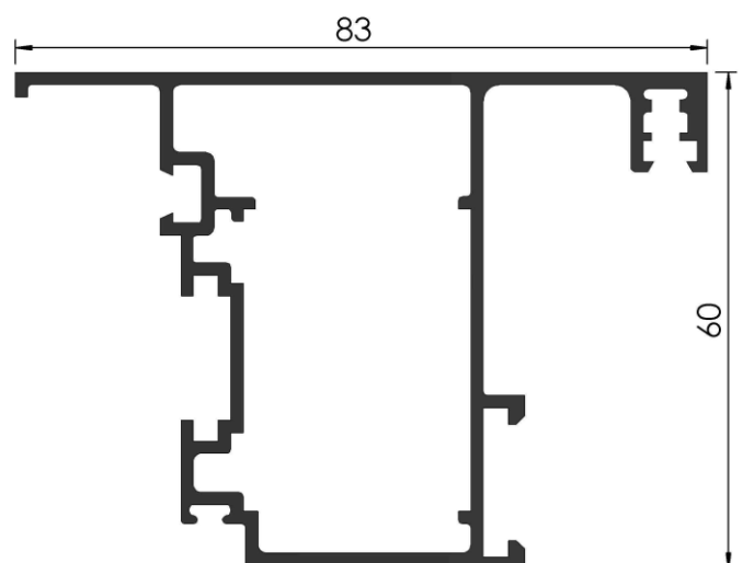
COD: RA 3/053 ENCUENTRO CENTRAL VENTANA DE ABRIR PESO: 1,094 Kg/m LARGO: 6200 mm.
