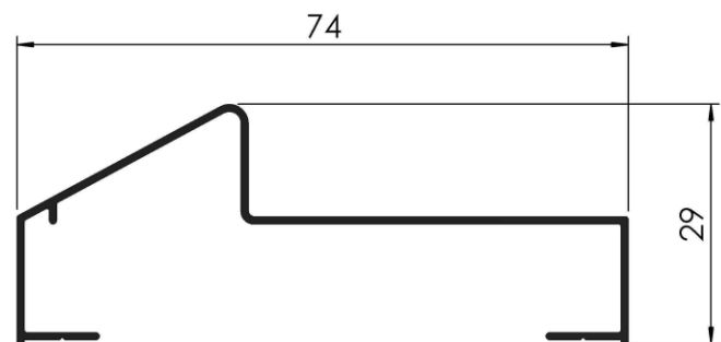
COD: RA E 1/479 MARCO DE PUERTA PLACA DE 2" ECONAL PESO: 0,350 Kg/m LARGO: 6200 mm.
