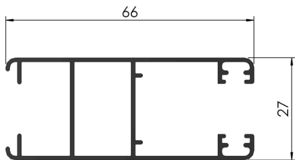
COD: RA / 261 HOJA CORREDIZA PESO: 0,673 Kg/m LARGO: 6030 mm.
