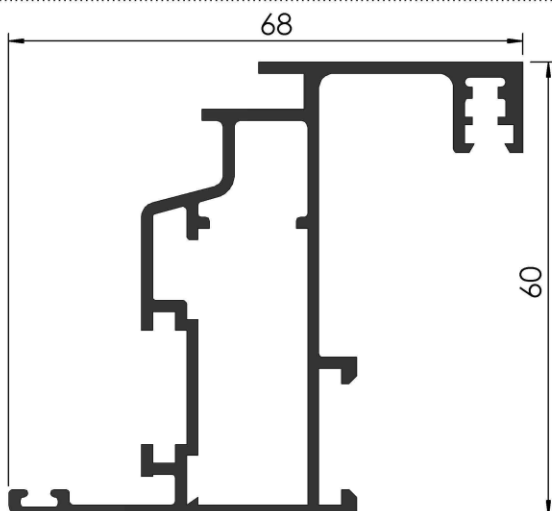
COD: RA 3/049 CONTRAVIDRIO RECTO LADO EXTERIOR PUERTA DE REBATIR PESO: 0,232 Kg/m LARGO: 6200 mm.
