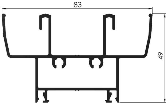
COD: RA 1/200 UMBRAL Y DINTEL MARCO VENTANA Y PUERTA CORREDIZA 90° PESO: 1,145 Kg/m LARGO: 6150 mm.
