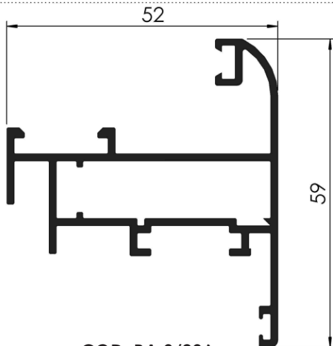
COD: RA 3/236 HOJA CURVA VENTILUZ PESO: 0,950 Kg/m LARGO: 6150 mm.
