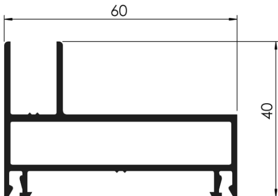
COD: RA 3/034 PARANTE LATERAL CORREDIZA PESO: 1,399 Kg/m LARGO: 6200 mm.
