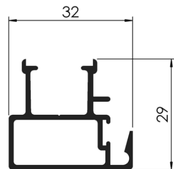
COD: RA 1/902 DINTEL UMBRAL PESO: 0,456 Kg/m LARGO: 6030 mm.
