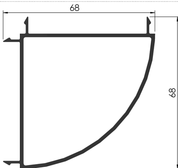
COD: RA 3/059 MARCO RECTO PAÑO FIJO Y VENTANA DE ABRIR PESO: 1,053 Kg/m LARGO: 6200 mm.
