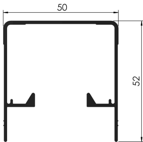
COD: RA 1/319 CABEZAL MAMPARA PESO: 0,715 Kg/m LARGO: 6030 mm.
