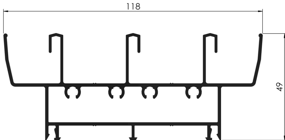
COD: RA 3/240 UMBRAL Y DINTEL MODENA 3 HOJAS 90° PESO: 1,700 Kg/m LARGO: 6150 mm.
