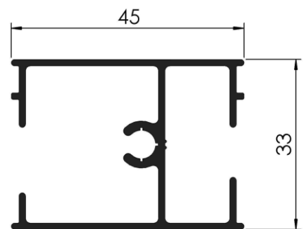
COD: RA 1/182 TRAVESAÑO ANGOSTO 36 mm. PESO: 0,620 Kg/m LARGO: 6030 mm.
