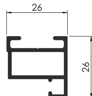
COD: RA 1/121 NÚCLEO DE VIDRIO REPARTIDO PESO: 0,360 Kg/m LARGO: 6030 mm.
