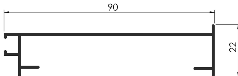
COD: RA 1/015 BISAGRA PROYECTANTE Y BANDEROLA PESO: 0,330 Kg/m LARGO: 6030 mm.
