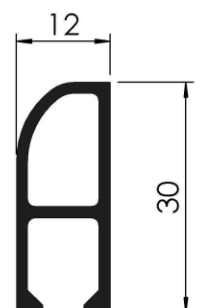
COD: RA 3/038 MOSQUITERO REFORZADO PESO: 0,594 Kg/m LARGO: 6200 mm.
