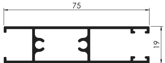
COD: RA 2/053 PARANTE LAT. PUERTA CORREDIZA REDONDEADO PESO: 0,760 Kg/m LARGO: 6150 mm.
