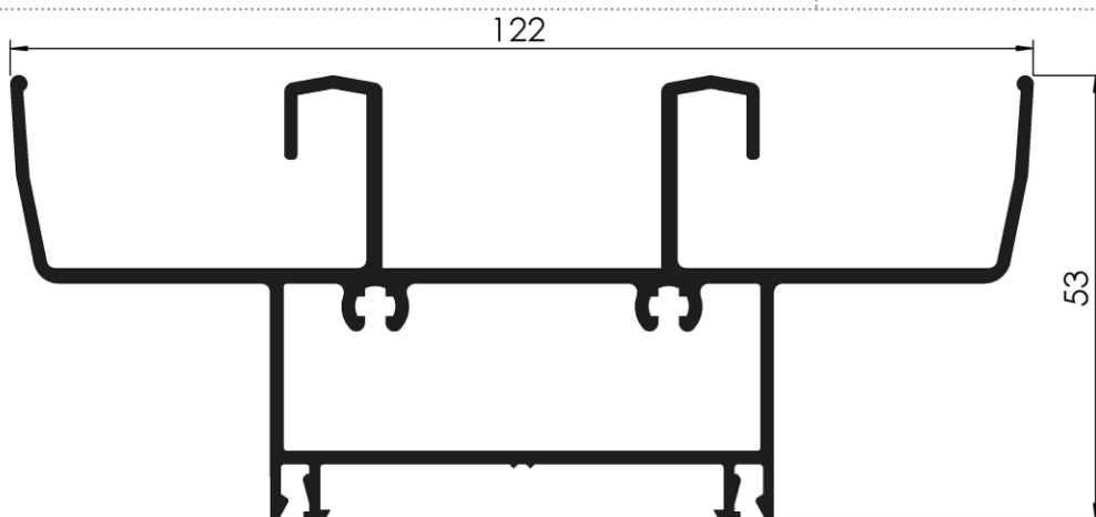
COD: RA 3/037 UMBRAL Y DINTEL DE MARCO PESO: 1,744 Kg/m LARGO: 6200 mm.
