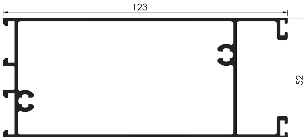
COD: RA 3/219 ZOCALO HOJA PUERTA DE REBATIR PESO: 1,658 Kg/m LARGO: 6030 mm.
