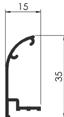
COD: RA 1/907 MARCO PAÑO FIJO PESO: 0,556 Kg/m LARGO: 6030 mm.
