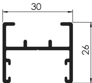
COD: RA 2/054 PARANTE CENT. PUERTA CORREDIZA REDONDEADO PESO: 0,685 Kg/m LARGO: 6150 mm.
