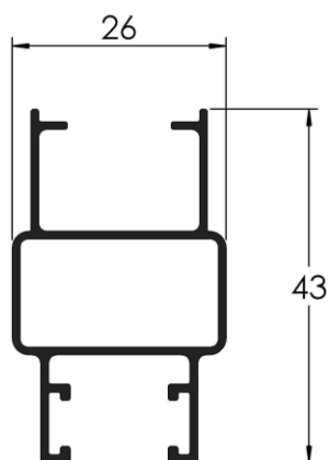
COD: RA E 1/903 PARANTE LATERAL HOJA PESO: 0,410 Kg/m LARGO: 6030 mm.
