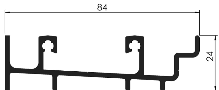
COD: RA 1/904 PARANTE CENTRAL HOJA PESO: 0,475 Kg/m LARGO: 6030 mm.
