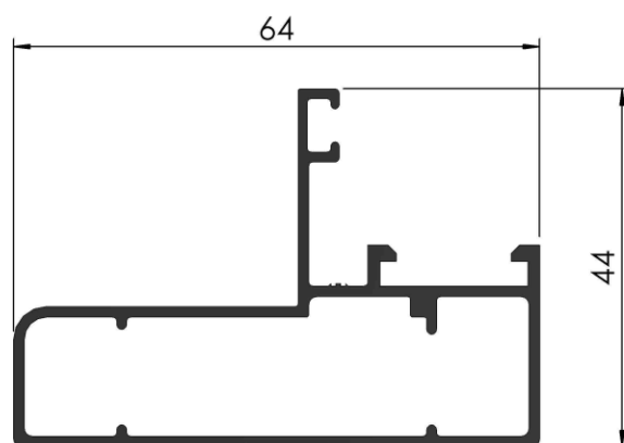
COD: RA / 160 MARCO ABRIR PESO: 0,777 Kg/m LARGO: 6150 mm.
