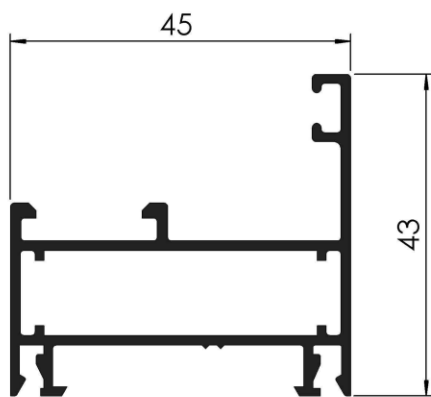
COD: RA 3/216 MARCO VENT. ABRIR BANDER. PUERTA REBATIR VENTILUZ PESO: 0,691 Kg/m LARGO: 6150 mm.
