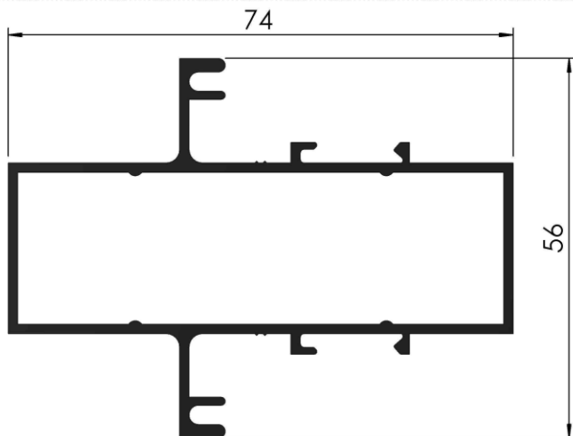
COD: RA 1/094 TRAVESAÑO PAÑO FIJO PESO: 0,980 Kg/m LARGO: 6030 mm.
