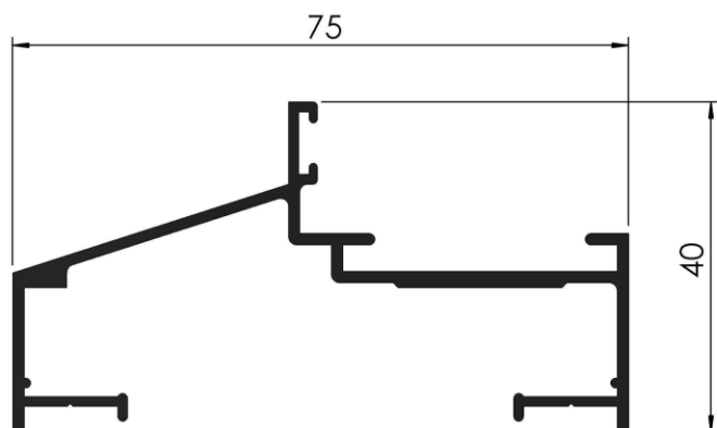
COD: RA 1/939 MARCO 36 mm. PESO: 0,676 Kg/m LARGO: 6200 mm.
