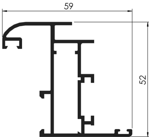
COD: RA 3/235 HOJA CURVA VENTANA DE ABRIR DC/BANDEROLA PESO: 0,905 Kg/m LARGO: 6150 mm.
