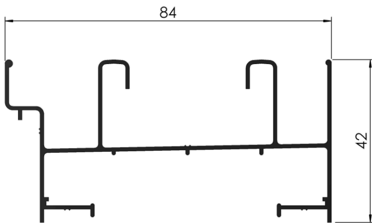
COD: RA 1/901 MARCO CORREDIZO PESADO PESO: 0,742 Kg/m LARGO: 6150 mm.
