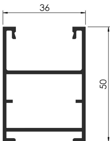
COD: RA 2/401 PARANTE POSTIGO REGULABLE PESO: 0,660 Kg/m LARGO: 6200 mm.
