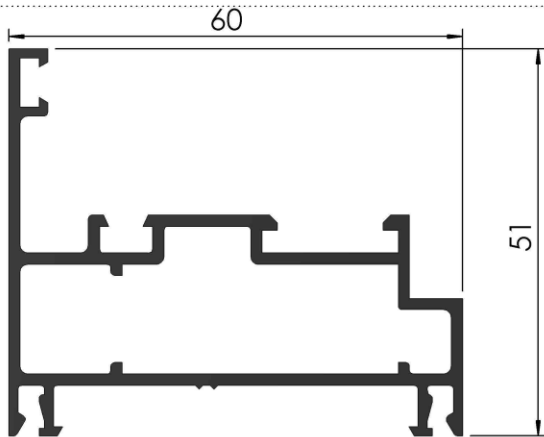
COD: RA 3/051 MARCO VENTANA DE ABRIR PESO: 0,986 Kg/m LARGO: 6200 mm.
