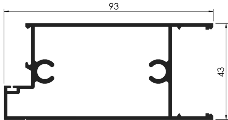
COD: RA 1/362 MARCO PUERTA 45 mm. PESO: 0,650 Kg/m LARGO: 6200 mm.
