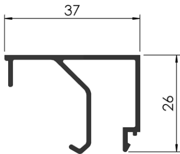
COD: RA 3/045 CONTRAVIDRIO RECTO P/VIDRIO SIMPLE PESO: 0,351 Kg/m LARGO: 6200 mm.
