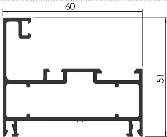
COD: RA 3/059 MARCO RECTO PAÑO FIJO Y VENTANA DE ABRIR PESO: 1,053 Kg/m LARGO: 6200 mm.
