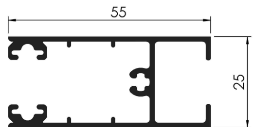
COD: RA 1/202 ZOCALO Y CABEZAL HOJA VENTANA CORREDIZA 90° PESO: 0,678 Kg/m LARGO: 6030 mm.
