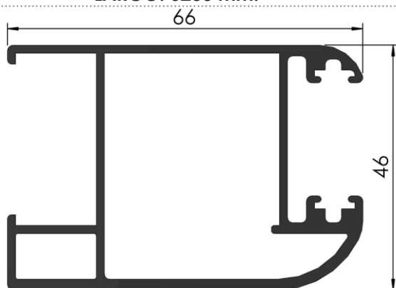
COD: RA 3/061 ZOCALO Y CABEZAL VENTANA CORREDIZA PESO: 0,942 Kg/m LARGO: 6200 mm.
