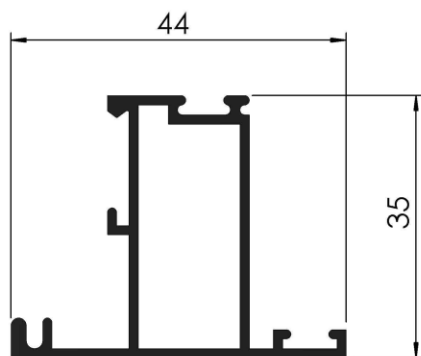
COD: RA 1/014 MARCO PROYECTANTE Y BANDEROLA PESO: 0,810 Kg/m LARGO: 6030 mm.
