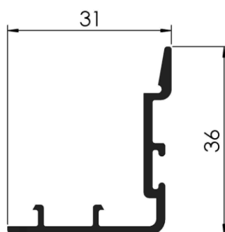
COD: RA 3/907 CLIP CIERRE MODENA 45° PESO: 0,334 Kg/m LARGO: 6150 mm.
