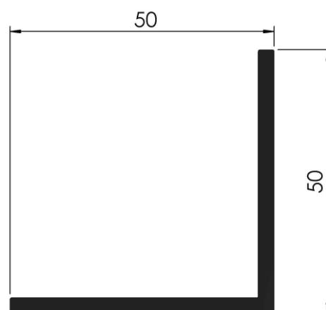
COD: RA 1/287 ANGULO 50 x 50 x 3 mm. PESO: 0,776 Kg/m LARGO: 6030 mm.
