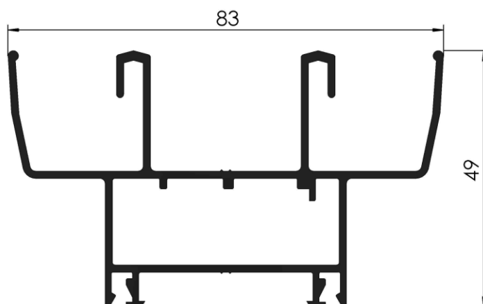
COD: RA 3/906 MARCO MODENA 45° PESO: 1,150 Kg/m LARGO: 6150 mm.
