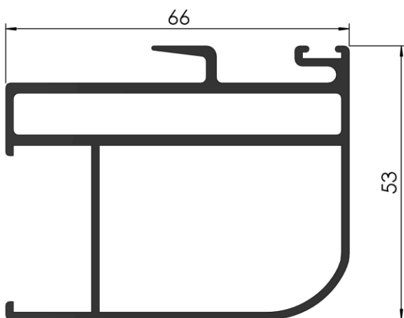
COD: RA 3/080 JAMBA DE MARCO CORREDIZA DE 3 HOJAS PESO: 1,701 Kg/m LARGO: 6200 mm.
