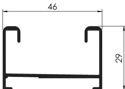
COD: RA 1/861 MARCO POSTIZO CORREDIZA PESO: 0,500 Kg/m LARGO: 6030 mm.
