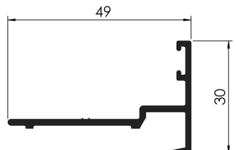
COD: RA 1/624 CABEZAL Y ZOCALO 45 mm. PESO: 1,310 Kg/m LARGO: 6030 mm.
