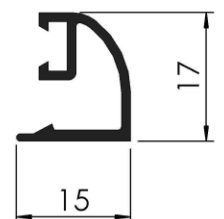
COD: RA 3/237 CONTRAVIDRIO EXTERIOR CURVO PUERTA DE REBATIR PESO: 0,175 Kg/m LARGO: 6030 mm.
