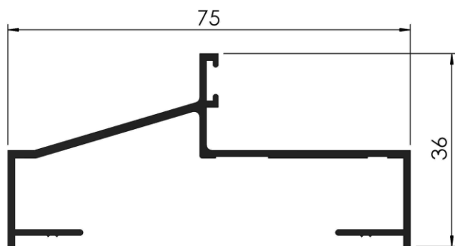
COD: RA 1/480 MARCO DE PUERTA PLACA DE 1 1/2" PESO: 0,590 Kg/m LARGO: 6200 mm.
