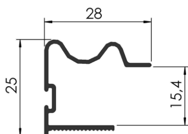
COD: RA / 4 MANIJA TIRADOR PLACARD PESO: 0,234 Kg/m LARGO: 6030 mm.
