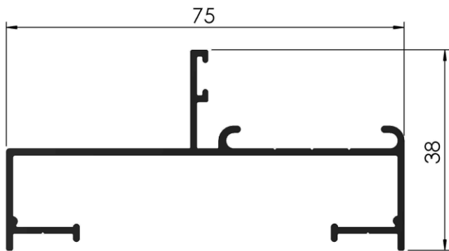
COD: RA 1/192 MARCO PUERTA RECTO 36 mm. PESO: 0,635 Kg/m LARGO: 6200 mm.
