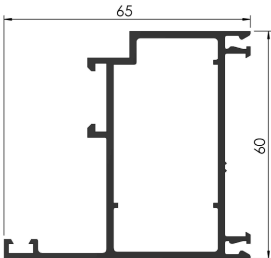
COD: RA 3/040 MARCO PUERTA DE REBATIR PESO: 1,180 Kg/m LARGO: 6200 mm.
