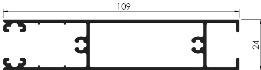
COD: RA 3/209 ZOCALO ALTO HOJA PARA VIDRIO SIMPLE PUERTA CORREDIZA PESO: 1,253 Kg/m LARGO: 6030 mm.
