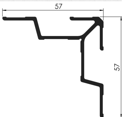
COD: RA 3/450 ESCUADRA DE ARMADO PESO: 0,605 Kg/m LARGO: 6030 mm.
