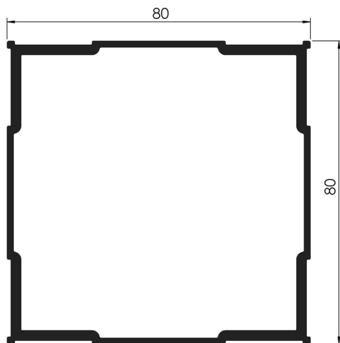
COD: RA 2/185 COLUMNA RECTA PESO: 1,453 Kg/m LARGO: 6150 mm.
