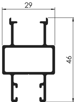
COD: RA 1/901 MARCO CORREDIZO PESADO PESO: 0,742 Kg/m LARGO: 6150 mm.
