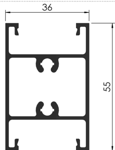
COD: RA 2/402 TRAVESAÑO POSTIGO REGULABLE PESO: 0,900 Kg/m LARGO: 6030 mm.
