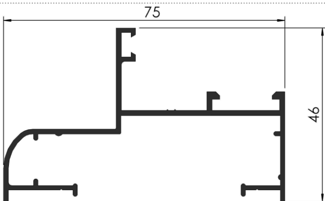
COD: RA 3/241 JAMBA 3 HOJAS CORREDIZA 90° PESO: 0,870 Kg/m LARGO: 6150 mm.
