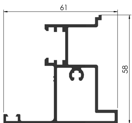
COD: RA 3/044 ENCUENTRO CENTRAL PUERTA DE REBATIR PESO: 1,037 Kg/m LARGO: 6200 mm.
