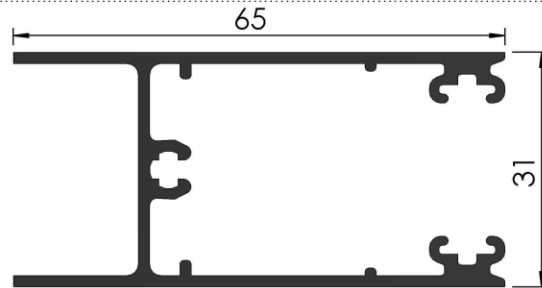
COD: RA 3/073 ZOCALO Y CABEZAL CORREDIZA P/DVH PESO: 0,861 Kg/m LARGO: 6200 mm.
