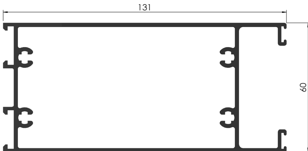
COD: RA 3/042 TRAVESAÑO PUERTA DE REBATIR PESO: 1,399 Kg/m LARGO: 6200 mm.
