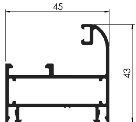
COD: RA 3/229 PAÑO FIJO CURVO PESO: 0,768 Kg/m LARGO: 6150 mm.
