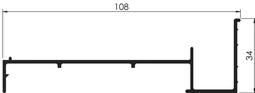
COD: RA 1/423 TABLILLA DE BARRIO TUBULAR PESO: 0,510 Kg/m LARGO: 6200 mm.
