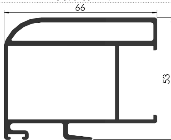
COD: RA 3/072 PARANTE CENTRAL CORREDIZA P/DVH PESO: 1,466 Kg/m LARGO: 6200 mm.
