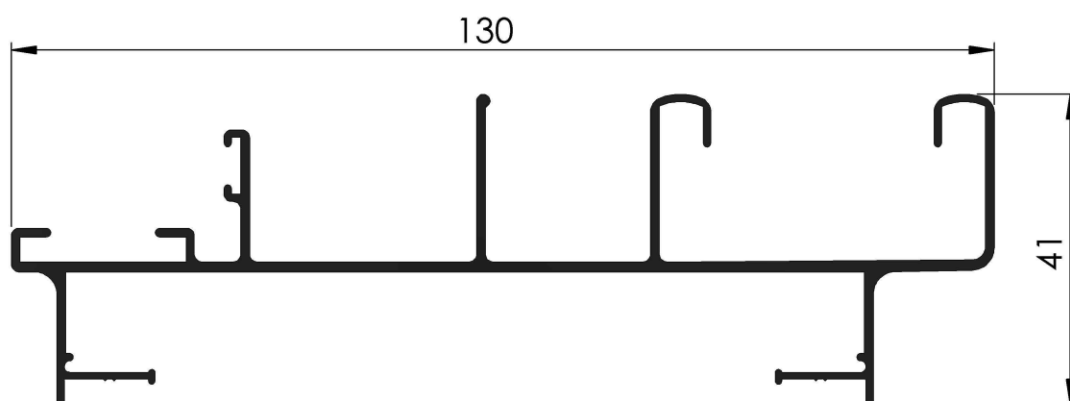
COD: RA 1/865 MARCO COMBINADO PESO: 1,062 Kg/m LARGO: 6030 mm.
