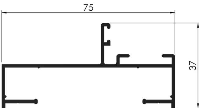
COD: RA 1/103 PARANTE DE CELOSÍA Y PUERTA LIVIANA PESO: 0,715 Kg/m LARGO: 6200 mm.
