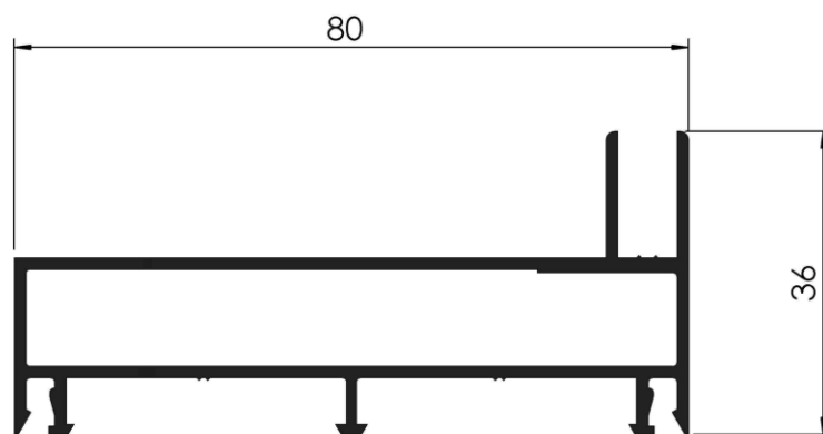
COD: RA 3/241 JAMBA 3 HOJAS CORREDIZA 90° PESO: 0,870 Kg/m LARGO: 6150 mm.
