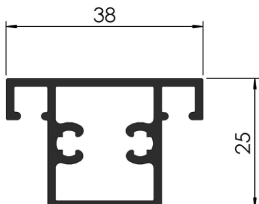
COD: RA 1/120 PERIMETRAL DE VIDRIO REPARTIDO PESO: 0,310 Kg/m LARGO: 6030 mm.
