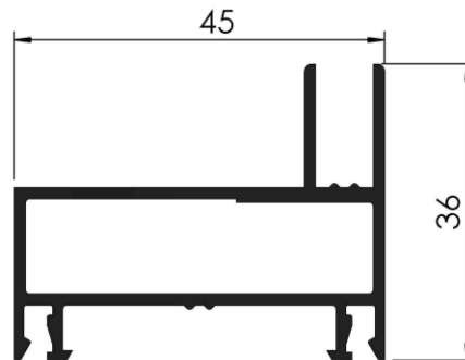
COD: RA 1/201 JAMBA DE MARCO DE VENTANA Y PUERTA 90° PESO: 0,665 Kg/m LARGO: 6150 mm.
