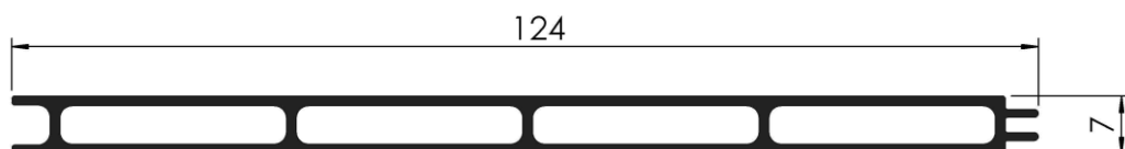
COD: RA 2/232 REVESTIMIENTO TUBULAR PESO: 1,039 Kg/m LARGO: 6030 mm.
