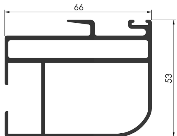
COD: RA 3/083 PARANTE CENTRAL TERCER HOJA PESO: 1,528 Kg/m LARGO: 6200 mm.
