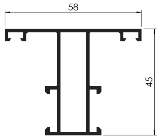
COD: RA 3/221 TRAVESAÑO ANGOSTO PAÑO FIJO PESO: 0,720 Kg/m LARGO: 6030 mm.
