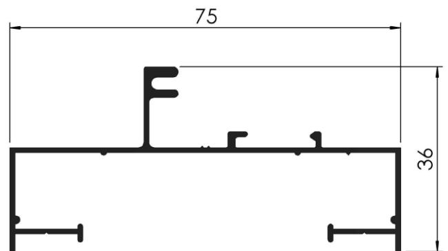
COD: RA 1/907 MARCO PAÑO FIJO PESO: 0,556 Kg/m LARGO: 6030 mm.
