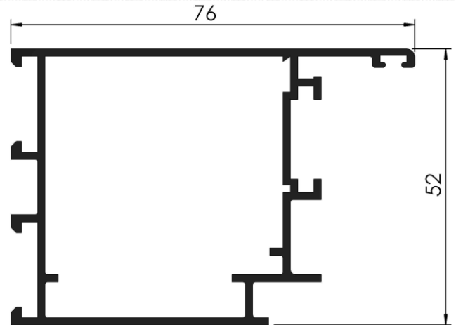
COD: RA 3/214 JAMBAS Y CABEZAL HOJA PUERTA DE REBATIR PESO: 1,085 Kg/m LARGO: 6200 mm.
